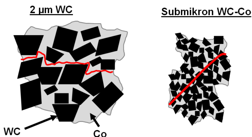
Obr. 2 – Mechanismus šíření trhliny v souvislosti s velikostí karbidického zrna[2] Fig. 2 – Crack propagation paths depending on the carbide grain size
